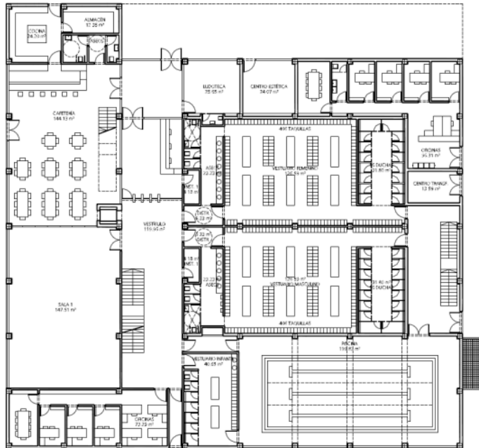
Planta baja
