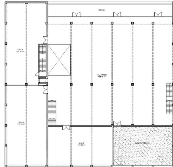
Planta alta
