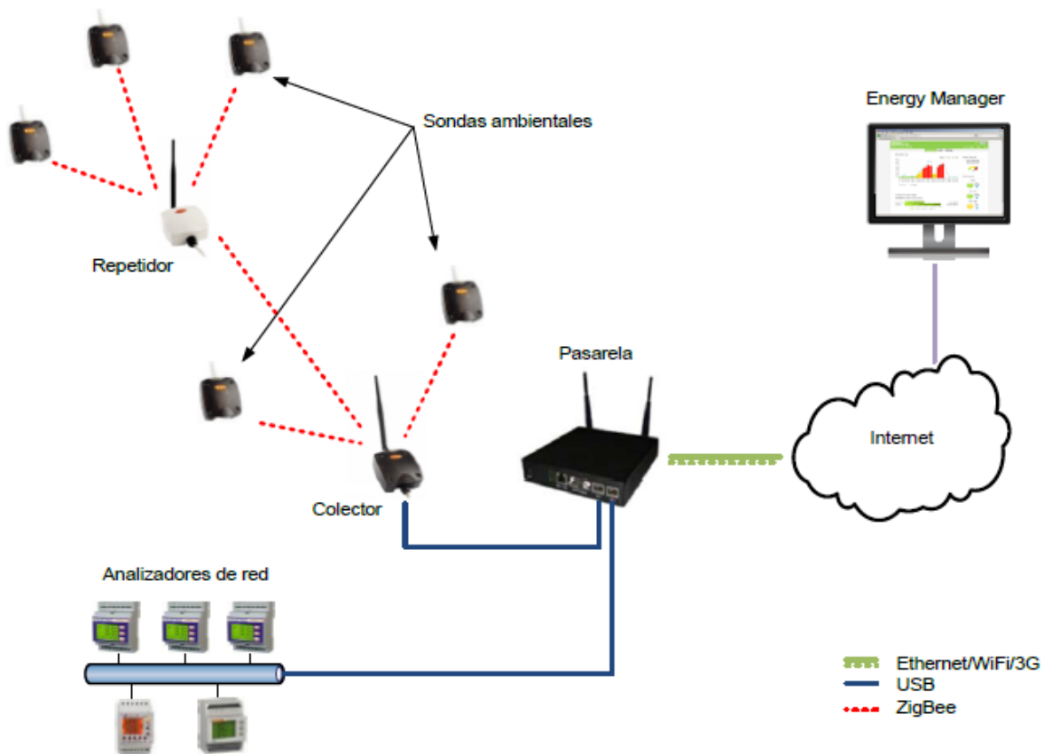
Arquitectura del sistema de monitorización
